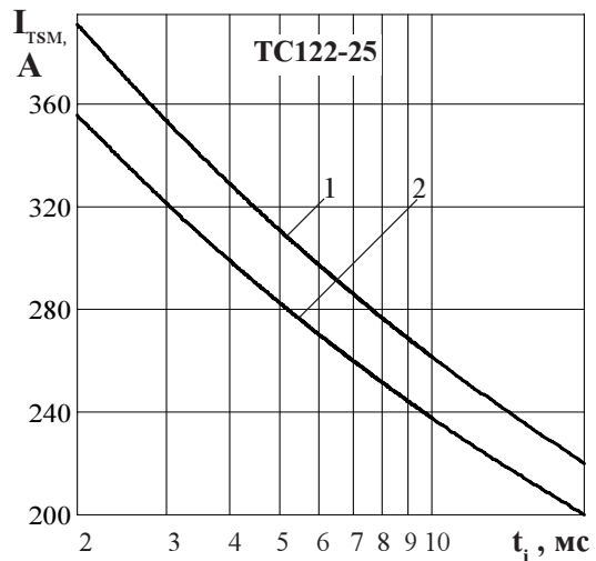
Рисунок 5 - Зависимость допустимой амплитуды ударного тока в открытом состоянии I_{TSM} от длительности импульса тока t_i при исходной температуре структуры T_j = 25^\circ C (1) и максимальной температуре T_{jm} (2)
