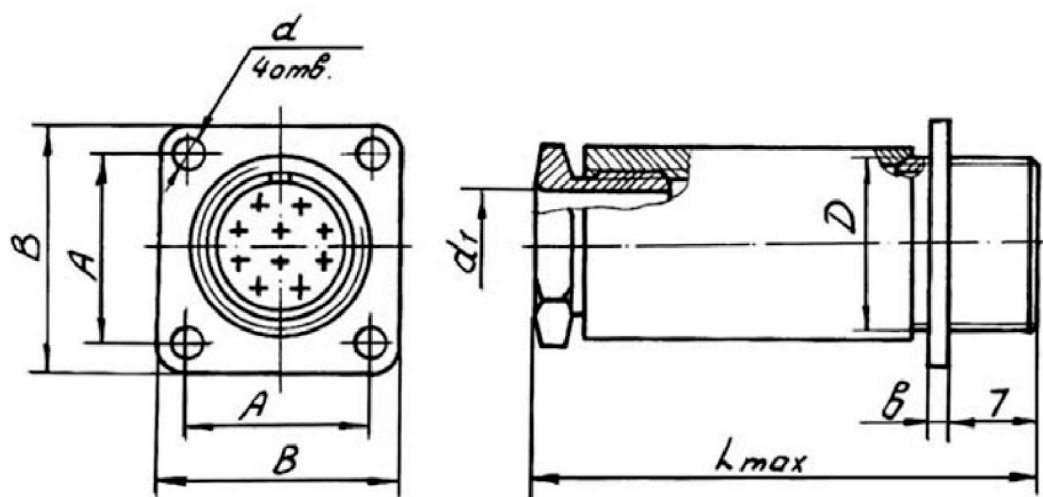
Вилка приборная РСТВ с кожухом:
