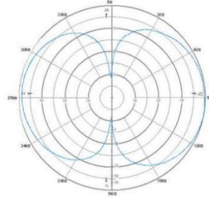
Vertical pattern 垂直方向图
