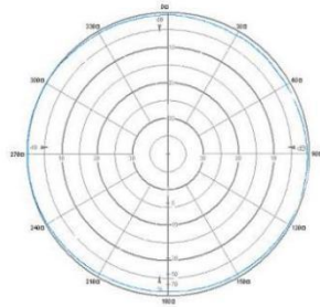
Horizontal pattern 水平方向图
