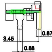
USB3.1 TYPE-C 02PF-023
